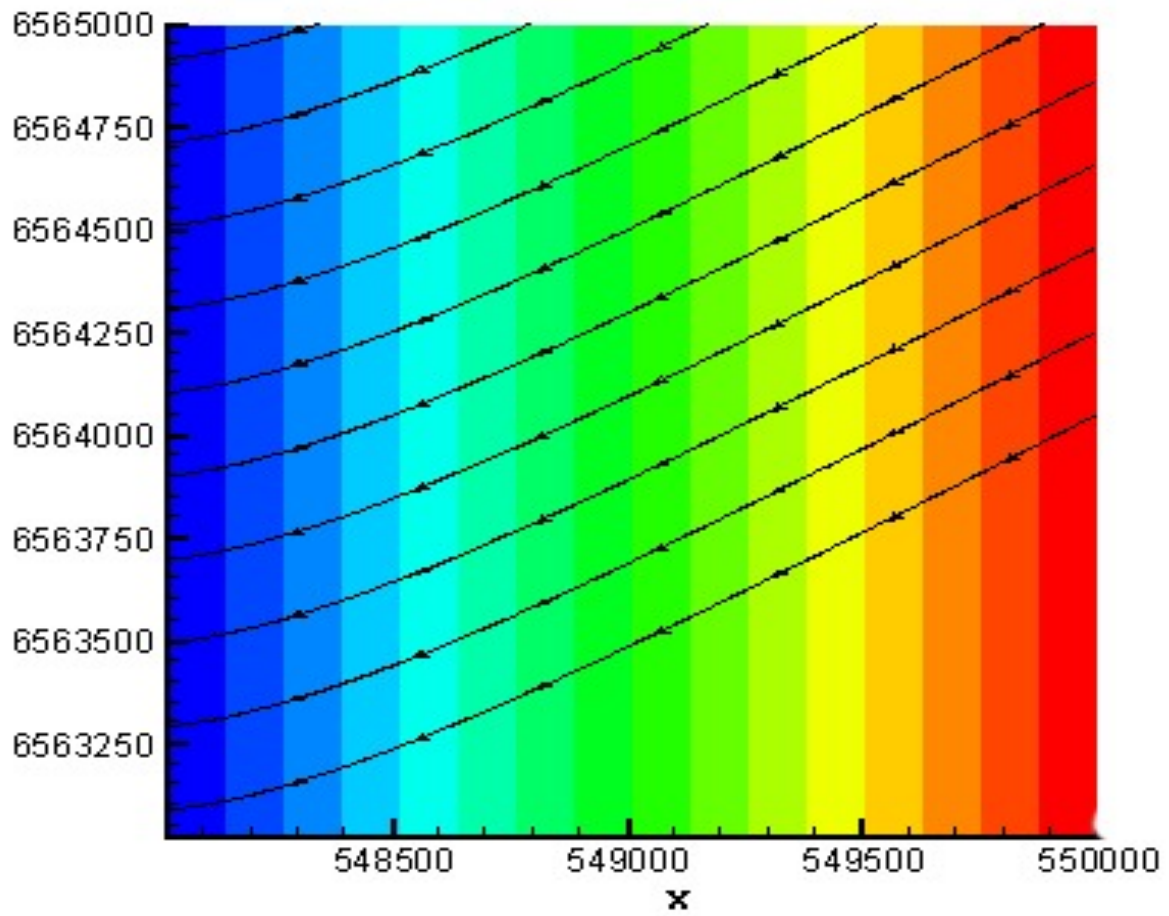
Figura 5. Raios de onda no exemplo rampa
